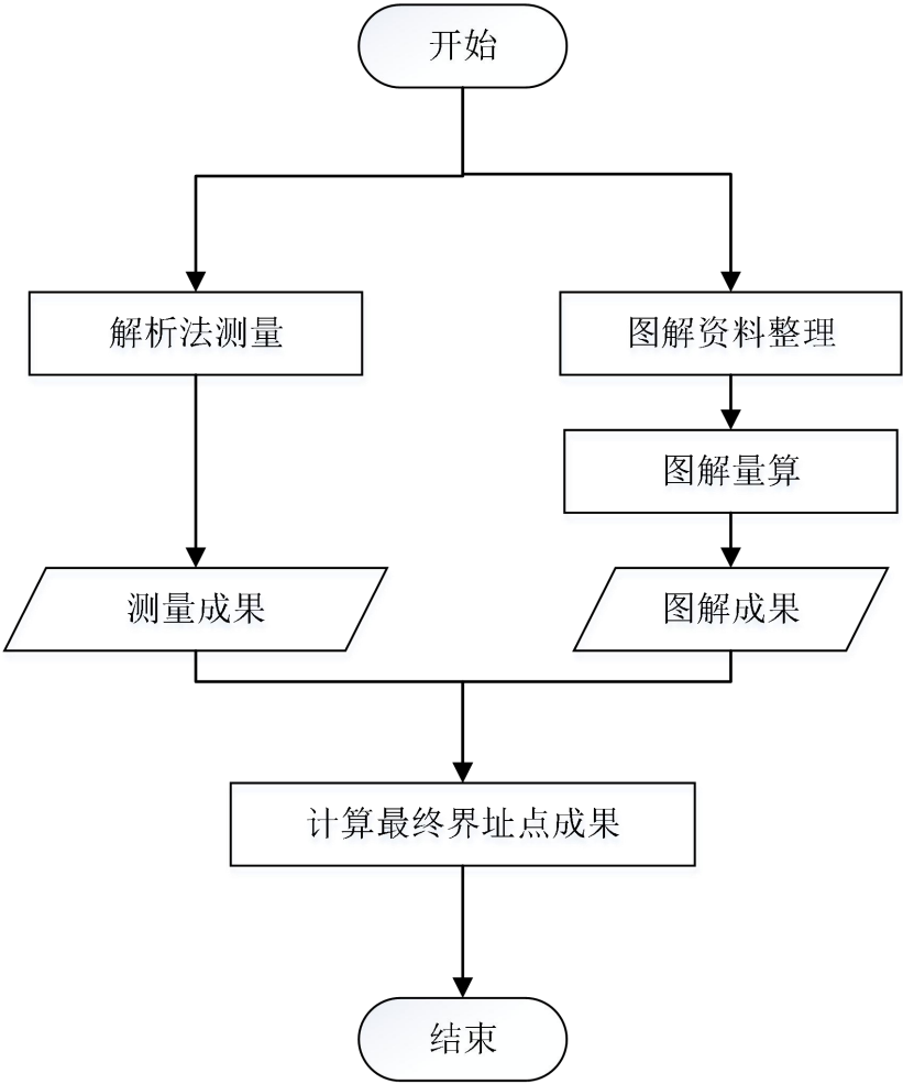
图 F.5 解析-图解法的界址点测量流程图
