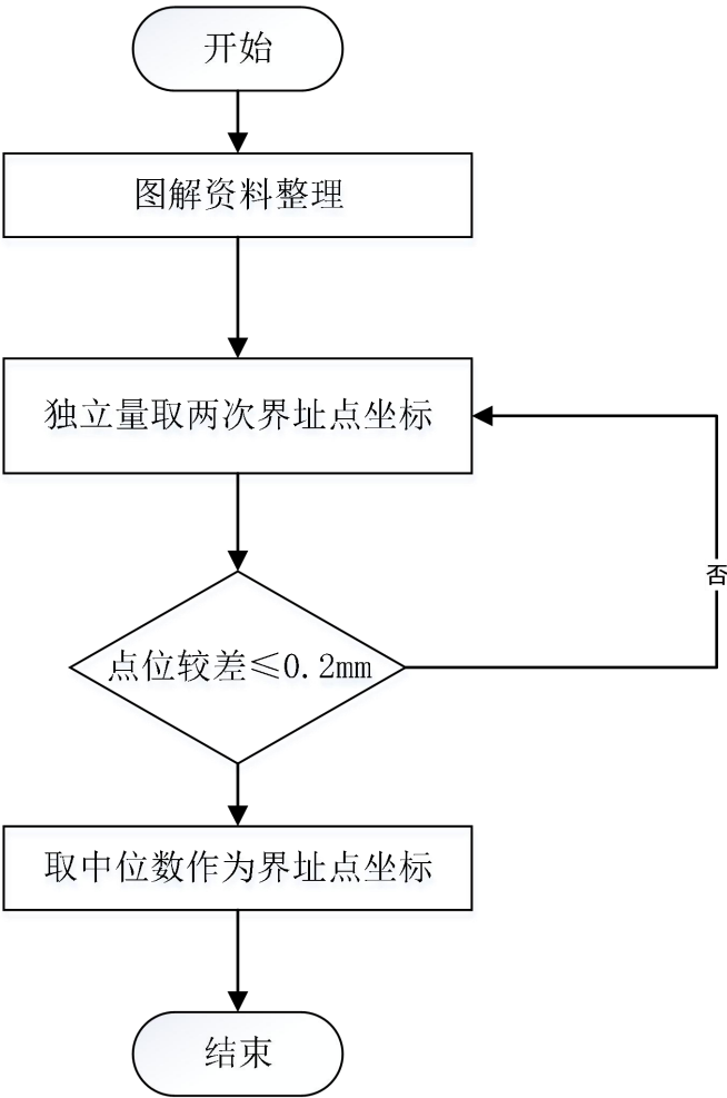
图 F.4 图解界址点流程图
