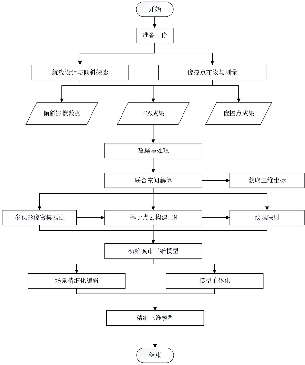
图 F.3 无人机倾斜摄影测量流程图
