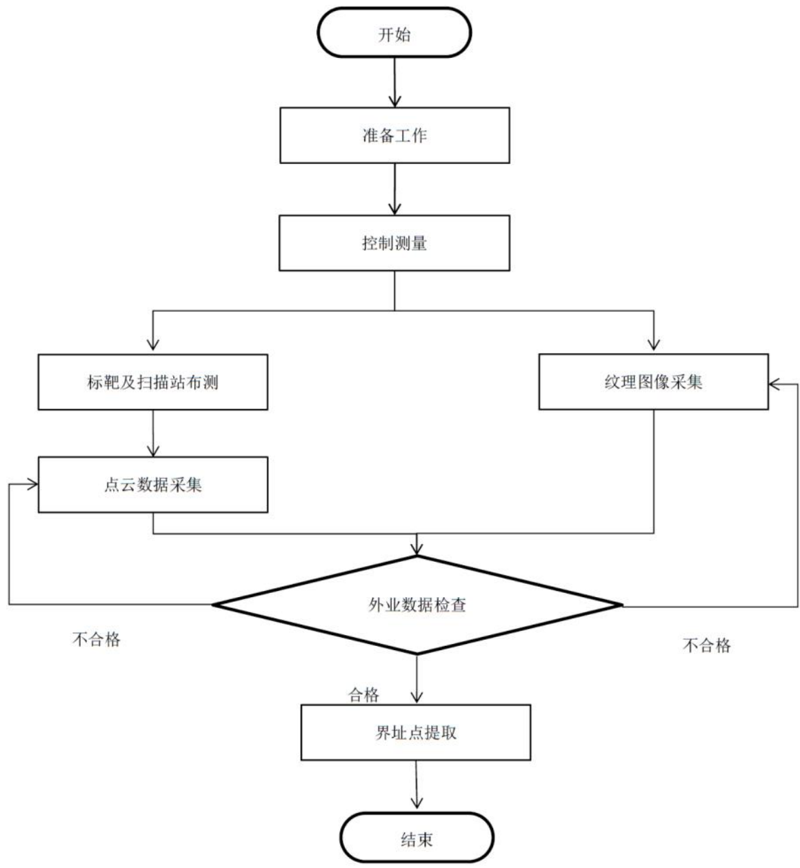
图 F.1 三维激光扫描测量流程图
