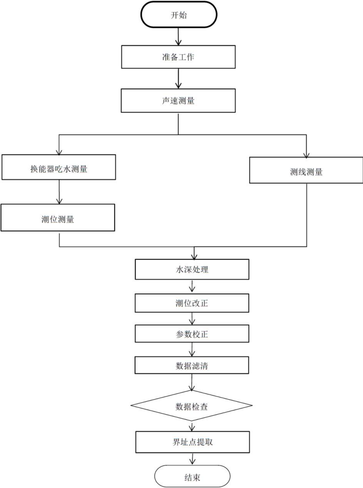
图 F.2 海洋多波束水深测量流程图海洋多波束水深测量流程图
