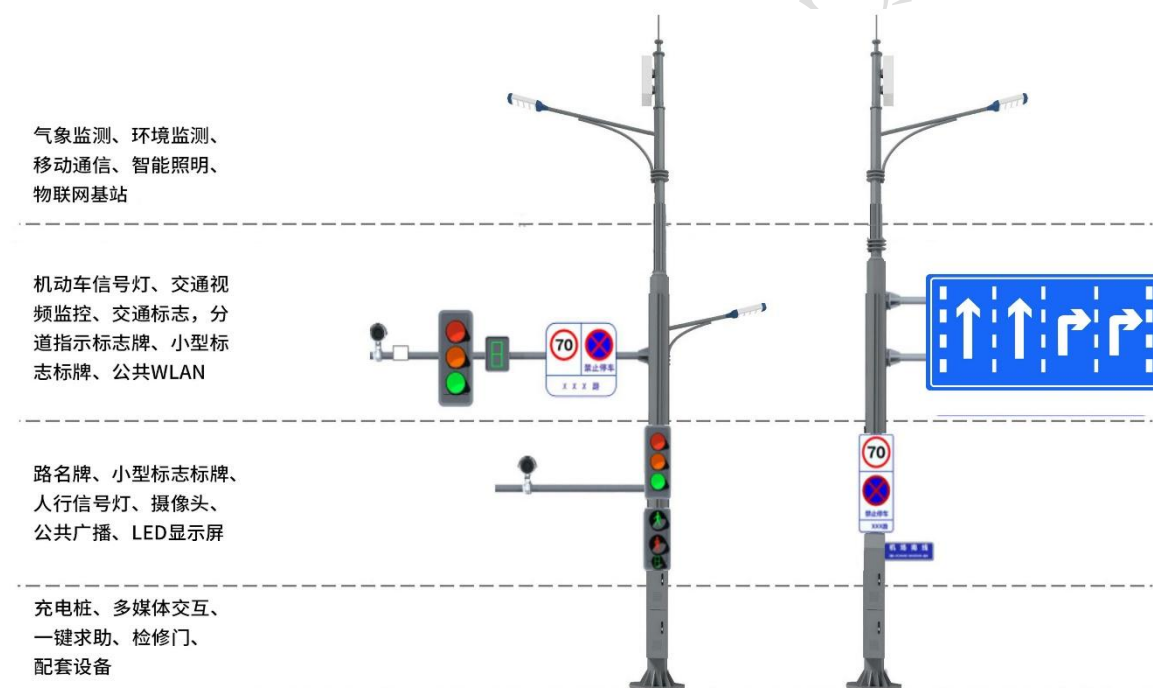
图 2 智慧灯杆分层设计示意图[DB4401/T 160—2022]
