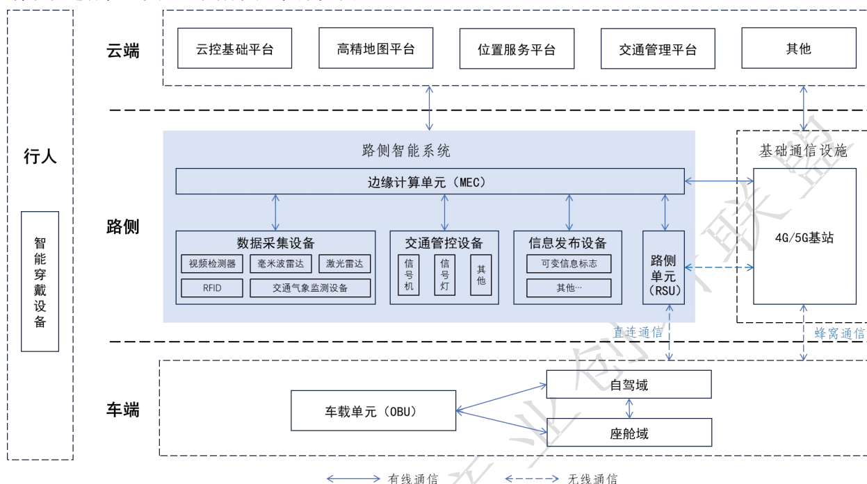
图 1 车路云一体化内部模块交互框架图
